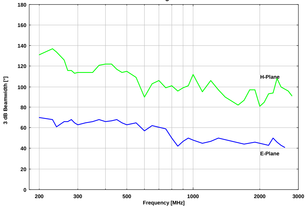
3 dB Öffnungswinkel:
