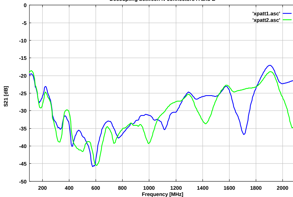
Entkopplung der Polarisations Ebenen A und B an den N-Buchsen Decoupling between N-connectors A and B
